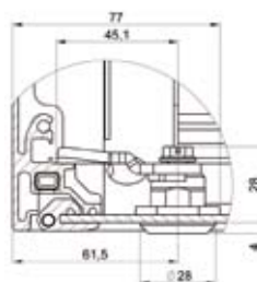
Vorreiberverschluss groß
