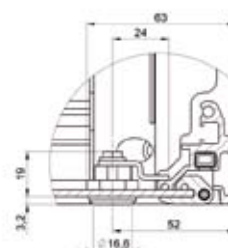
Vorreiberverschluss klein
